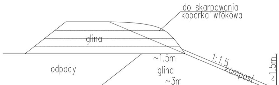
Schemat 1. Wbudowywanie odpadów w korpus składowiska metodą wałków prowadzących.
