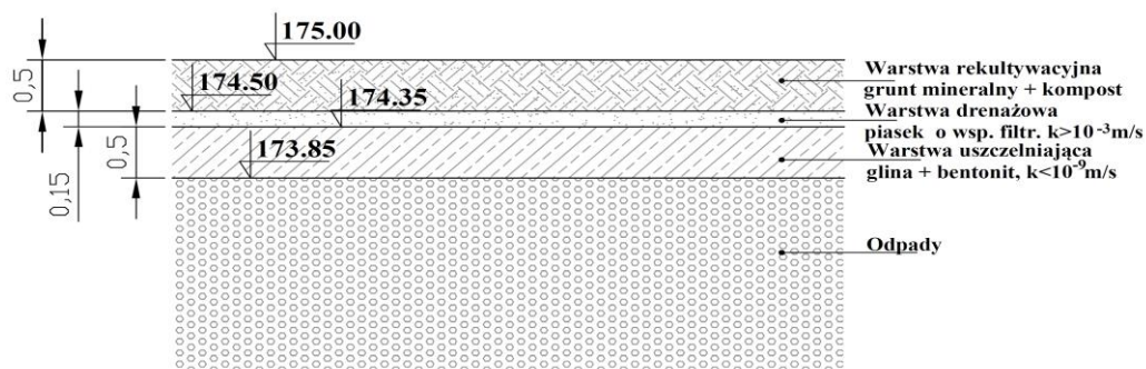
Schemat 2. Przykrycie mineralne powierzchni składowiska.
