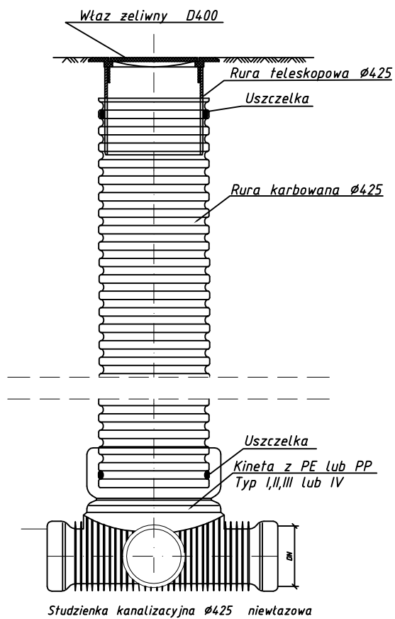
Studzienka kanalizacyjna Ø425 niewentylowana
