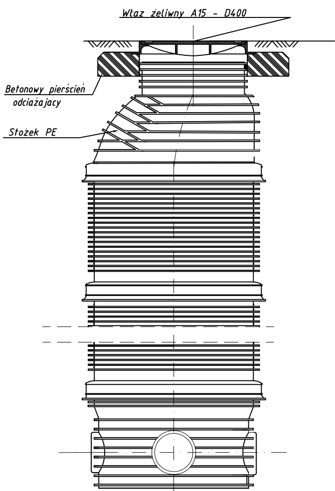
Studzienka kanalizacyjna TEGRA 1000
